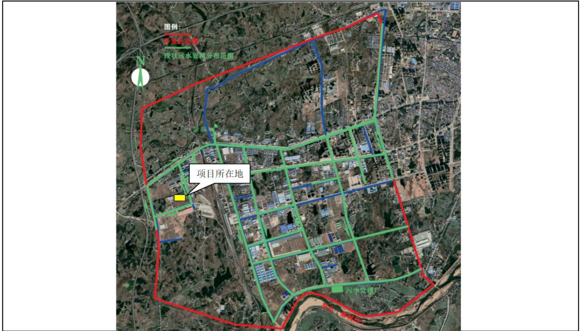
附图7 麻城经济开发区（2020年）现状污水管网分布图
