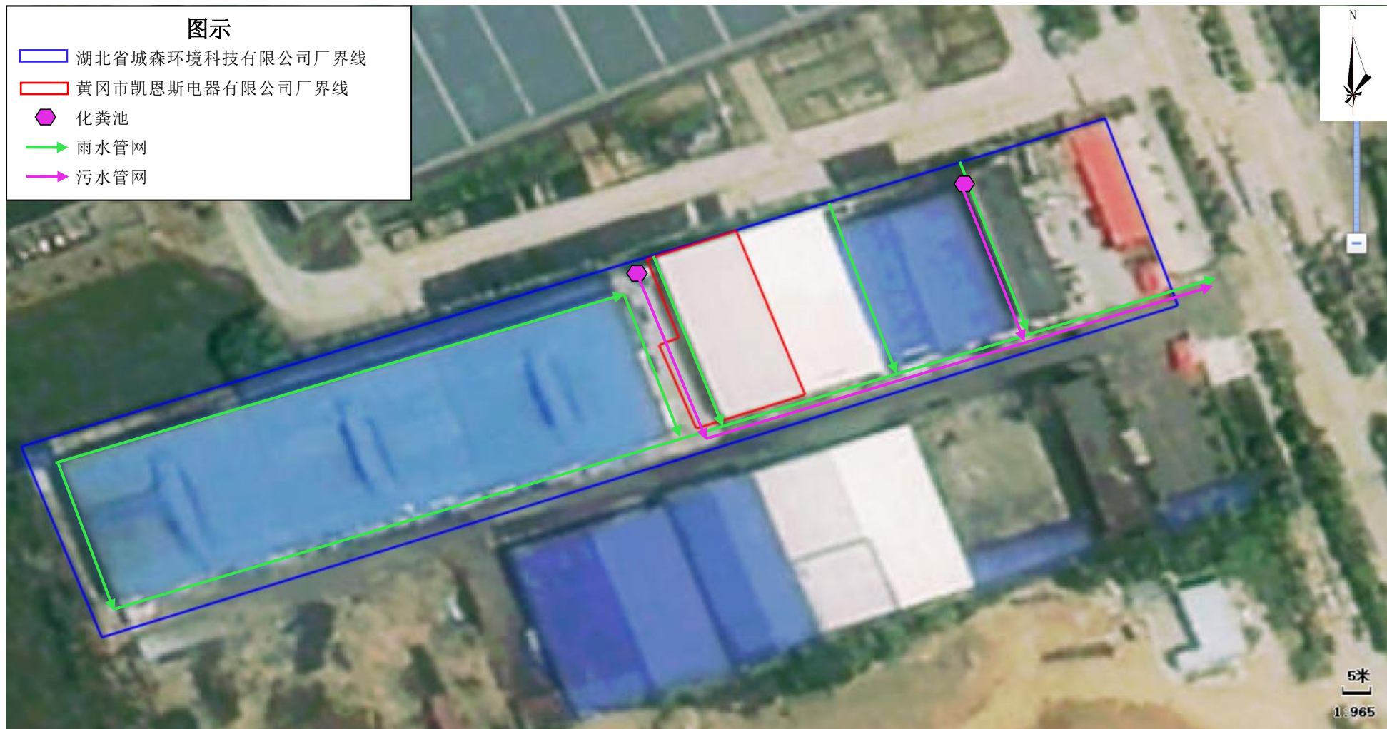
附图5 雨污管网图
