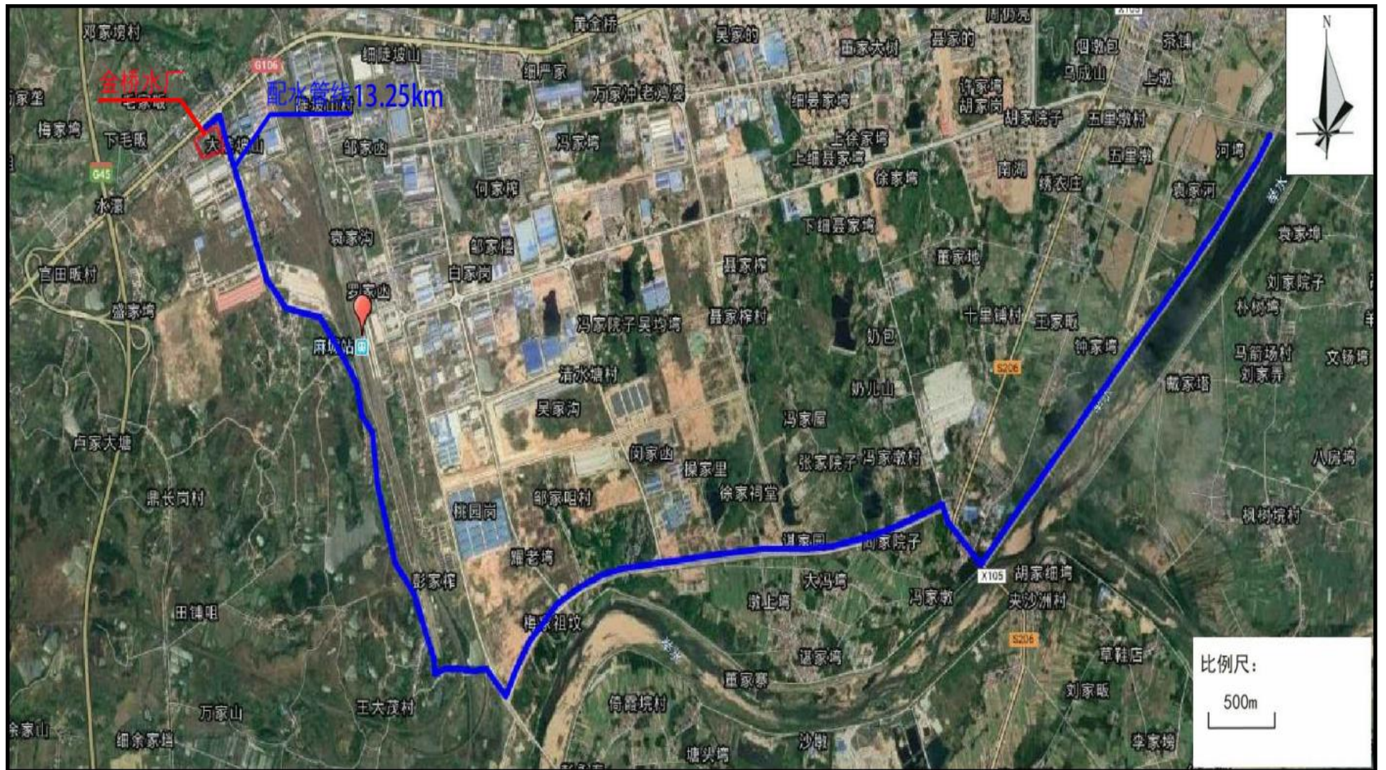
附图 2 项目总体范围配水管线示意图
